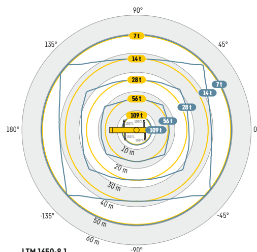
LTM 1650-8.1 54 m 100% 109 t 65 t
